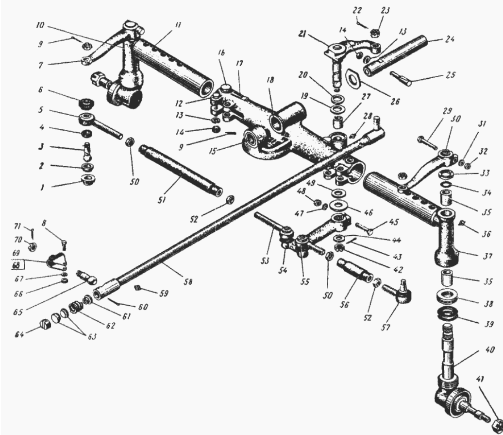
Рис. 38. Передняя ось и поворотные кулаки. Рулевые тяги
